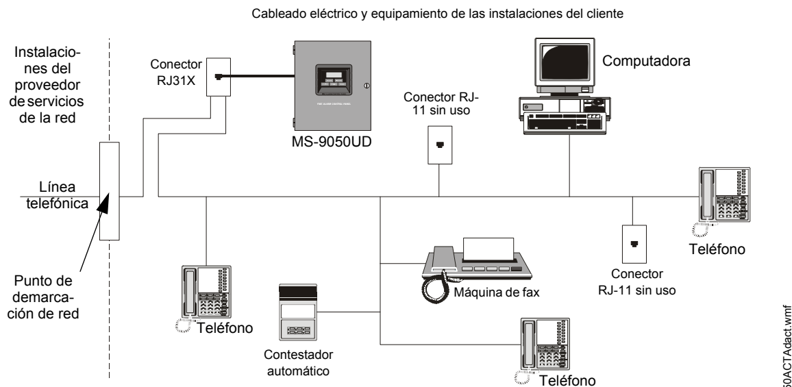
Figura 2.8 Instalación del DACT
