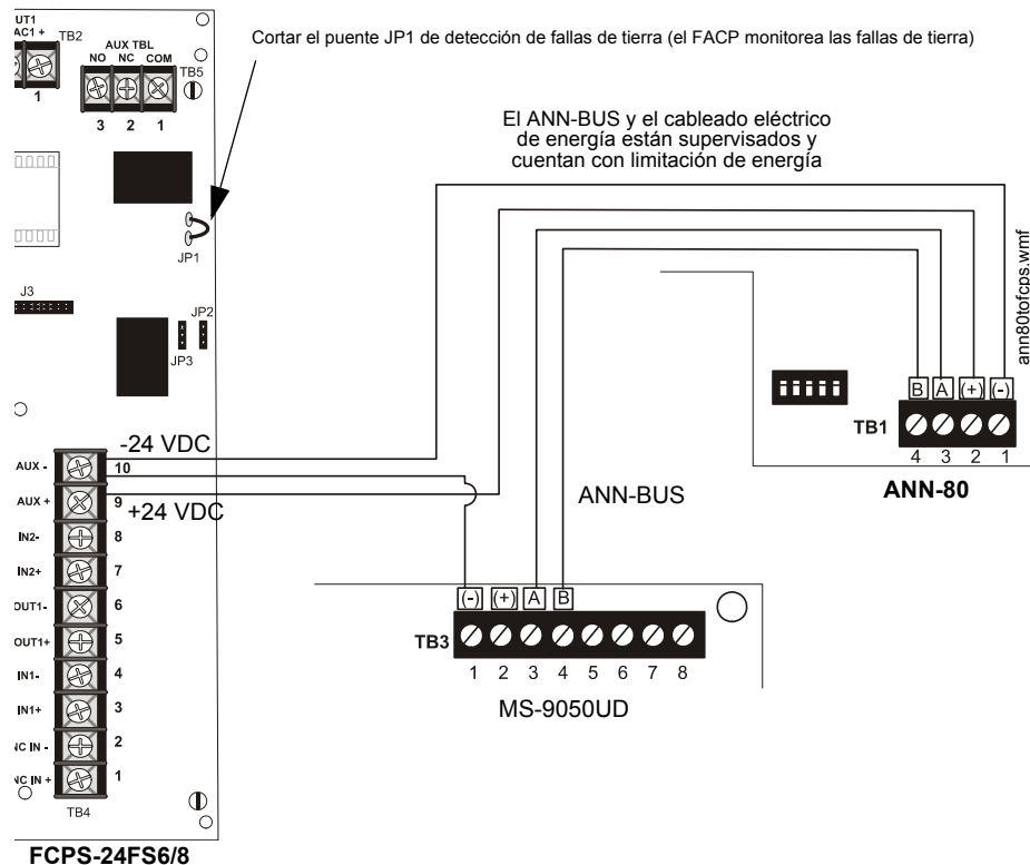
Figura 2.14 Provisión de energía de dispositivos ANN-BUS desde FCPS-24FS6/8
