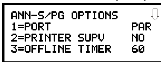
Pantalla Opciones ANN-S/PG #1
