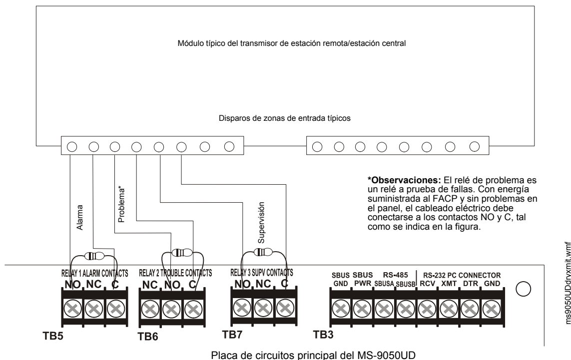
Figura C.4 Conexión de los contactos estacionarios del FACP al transmisor de la estación remota/estación central.
