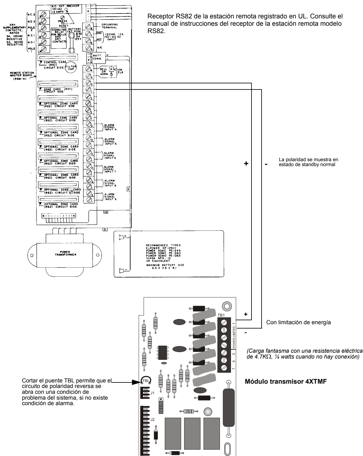
Figura C.2 Conexión con la estación remota mediante el módulo 4XTMF
