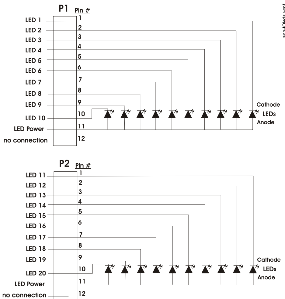
Figura 2.19 Cableado eléctrico de luces LED de ANN-I/O
