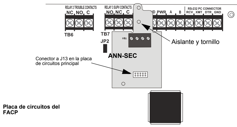
Figura 2.12 Instalación de la tarjeta de opciones ANN-SEC
